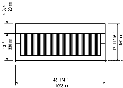
Bočna/o
